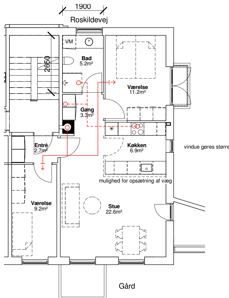
Fremtidig 1 : 100
