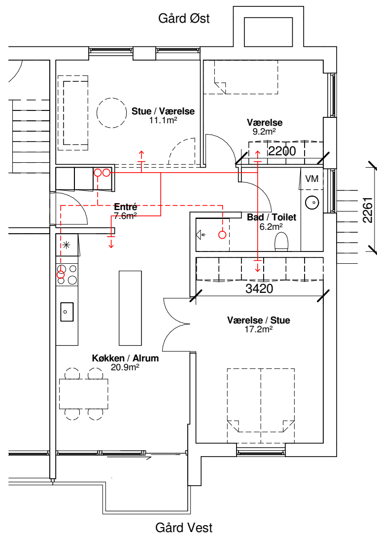
Fremtidig 1 : 100
